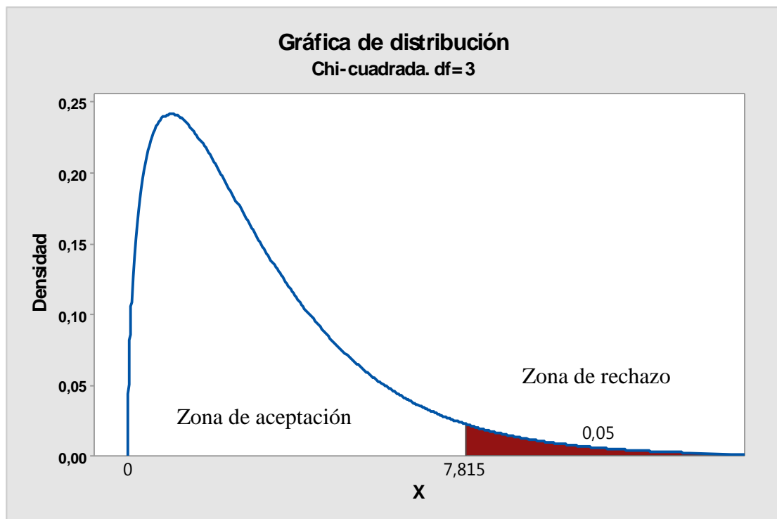
Gráfico N°27: Gráfica de distribución Chi-cuadrada Elaborado por: Fernanda Viteri
