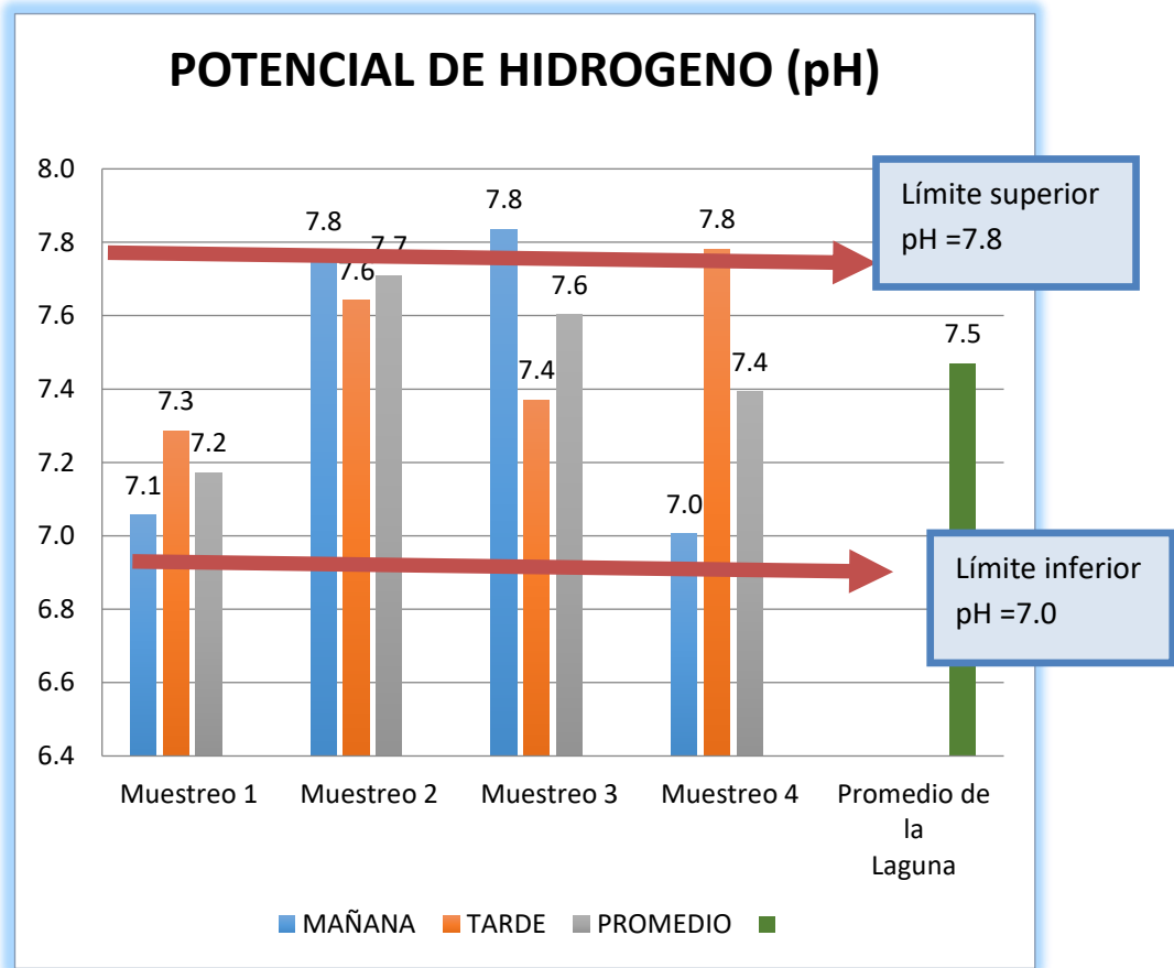
Gráfico 10: Resultados pH de 48 muestras de 6 puntos de la Laguna del Quilotoa Diciembre 2018-Enero 2019 frente a valores de referencia de la Norma de Calidad Ambiental y de Descarga de Efluentes: Recursos Agua.
