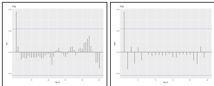
Figura 6: FN3 - ACF, PACF
