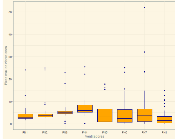
Figura 3: Diagrama de caja de los FNs
