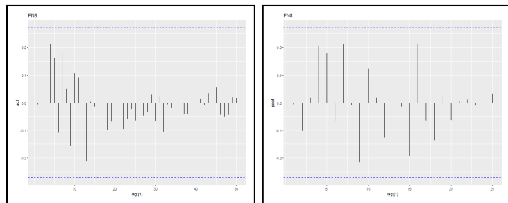
Figura 10: FN7 - ACF, PACF
