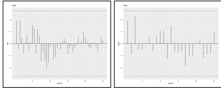
Figura 8: FN5 - ACF, PACF
