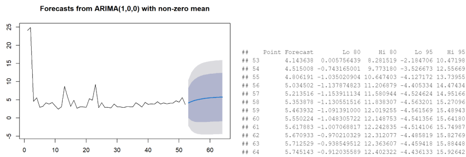
Figura 17: Pronósticos para FN2
