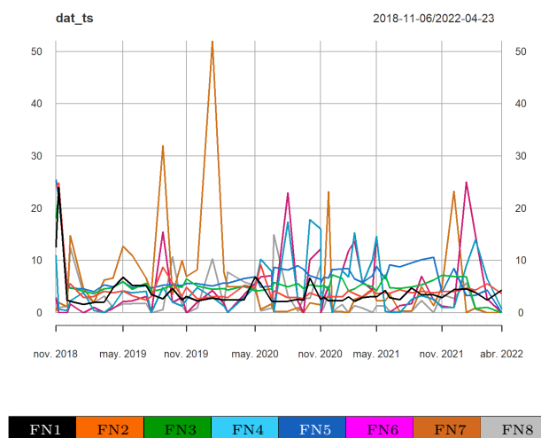
Figura 2: Series de tiempo de vibraciones máximas - FNs
