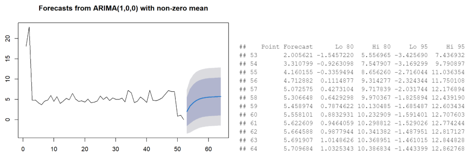
Figura 18: Pronósticos para FN3
