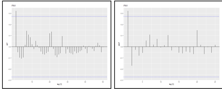
Figura 4: FN1 - ACF, PACF
