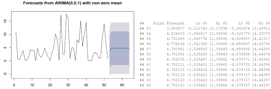
Figura 20: Pronósticos para FN5
