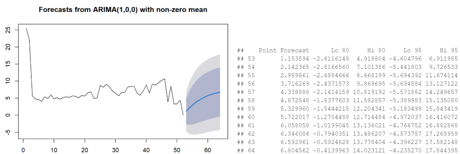
Figura 19: Pronósticos para FN4
