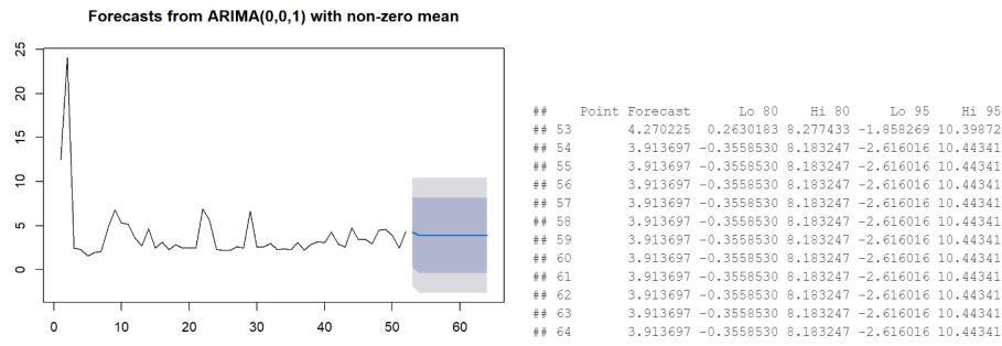
Figura 16: Pronósticos para FN1
